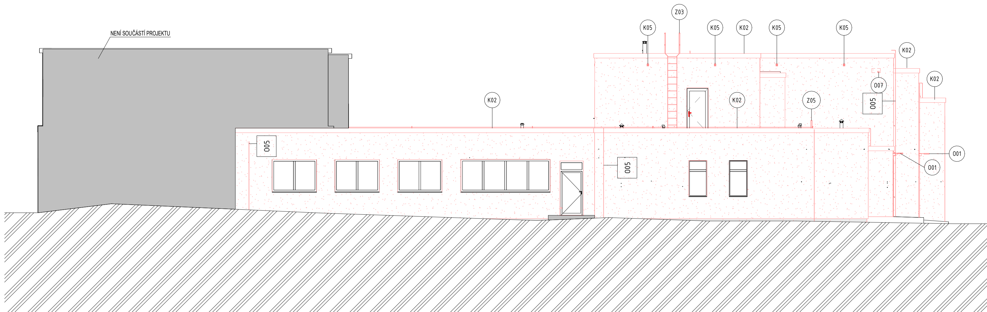
Pohled "V" - východní, M 1:100
